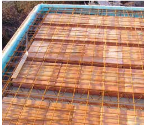
Obr. 1.14 Stropní konstrukce s výplní z keramických vložek
