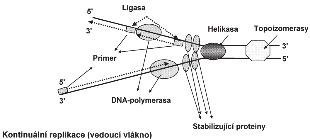
Obr. 7.5 Replikace DNA
