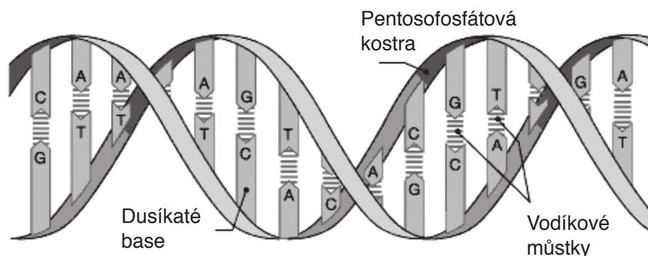
Obr. 7.2 Dvoušroubovice DNA
