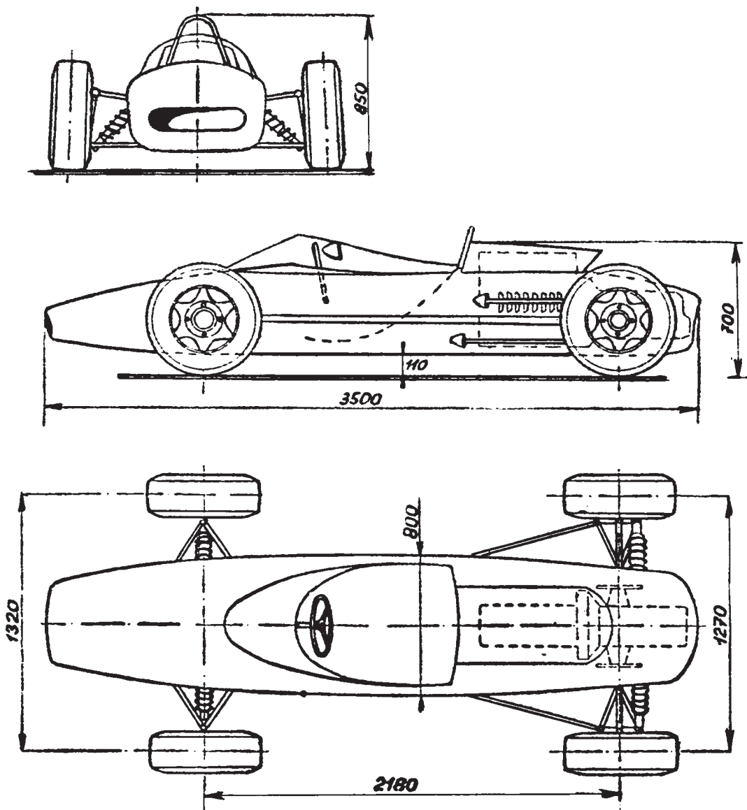
Rozměrový náčrt Šustova vozu F3 s motorem Ford, 1962–68
