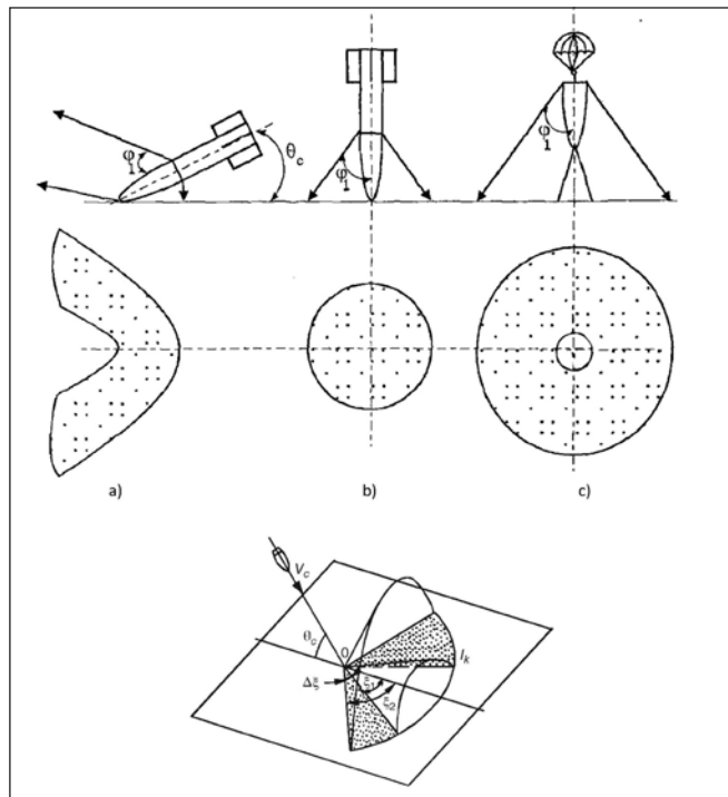
Obr. 1-11: Distribuce fragmentů bojové hlavice: a) dopad pod úhlem; b) vertikální dopad; c) vertikální dopad s aktivací distančním zapalovačem (nahore a uprostřed). (Zdroj: A. P. Orlov, Osnovy ustrojenia i funkcionirovania snarjadov RSZO ); vytváření sektorů ničivého účinku na povrchu země (dole). (Zdroj: I. Balagansky, Damaging Effects of Weapons and Ammunition )
