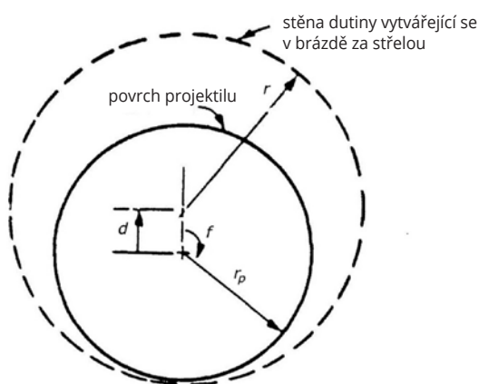
Pohled zezadu v podélné ose na průřez projektilu
