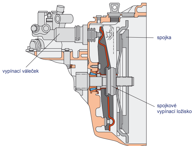
Princip fungování spojky
