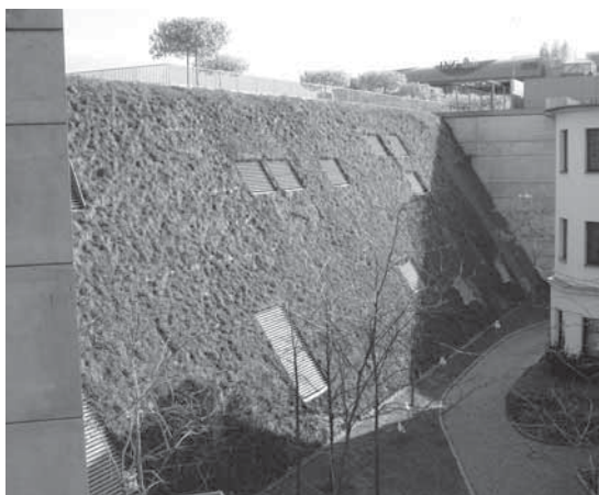
Obr. 1.15 KOC Nový Smíchov, strmá střeška o sklonu 58°, Praha 5, rok 2006
