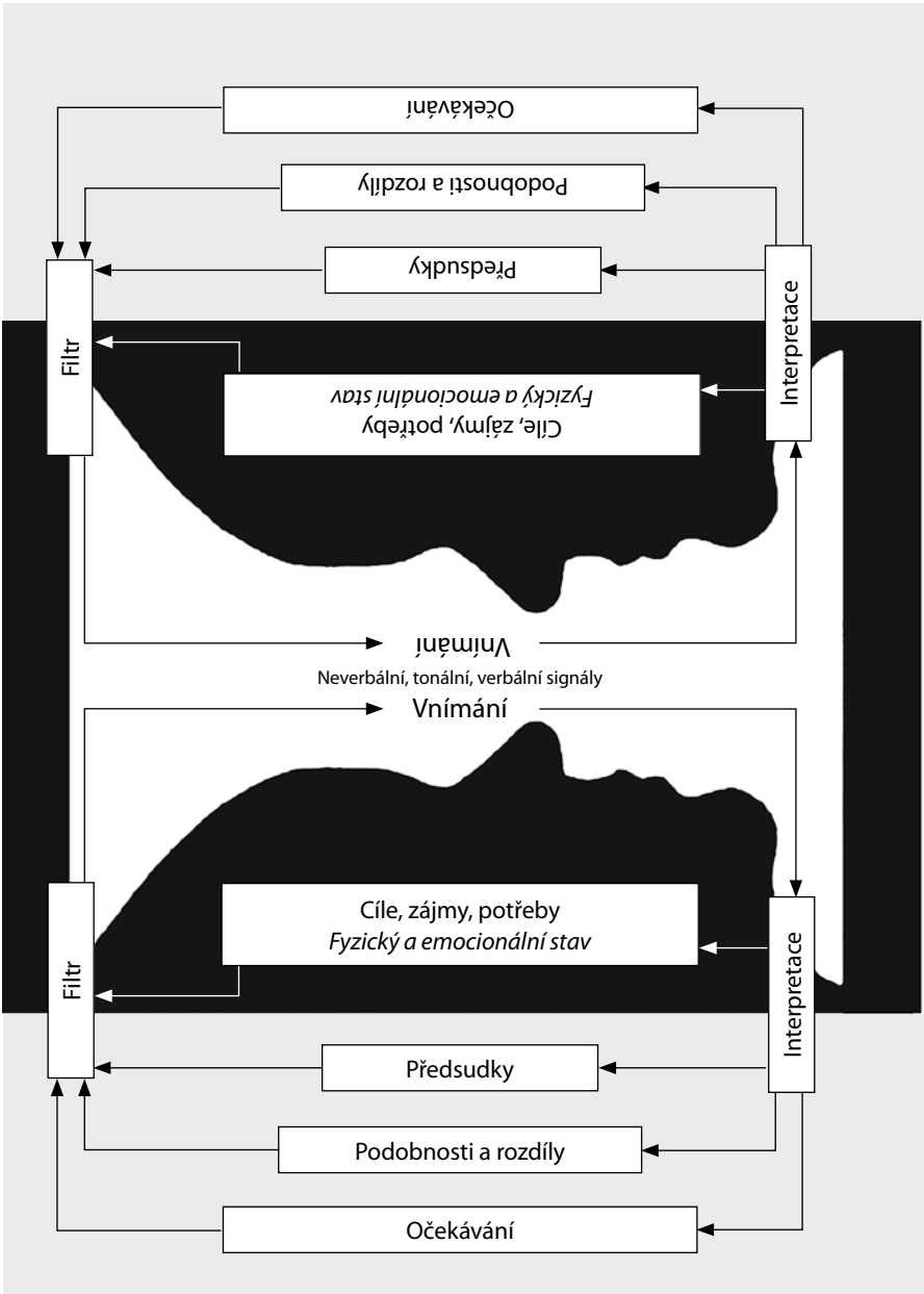
Obr. 1: Proces komunikace
