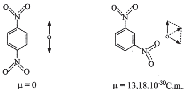
Obr. 1.3. Příklad znázornění vektorového součtu skupinových momentů
