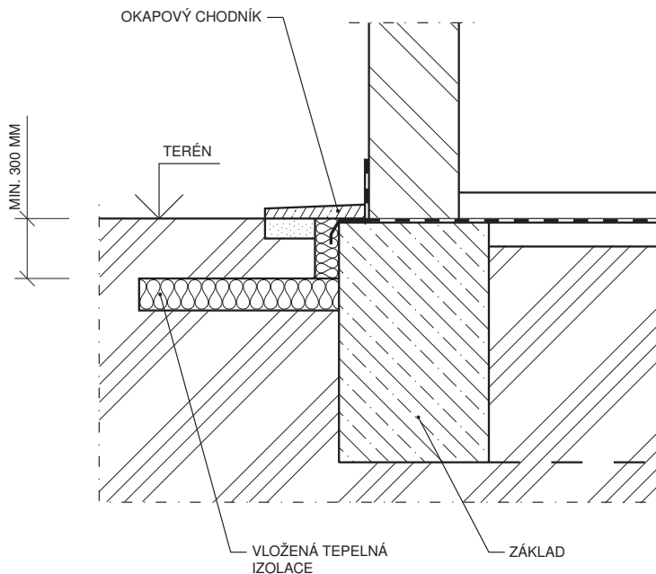
Obr. 5 Dosažení potřebné nezámrazné hloubky vložení tepelné izolace do terénu
