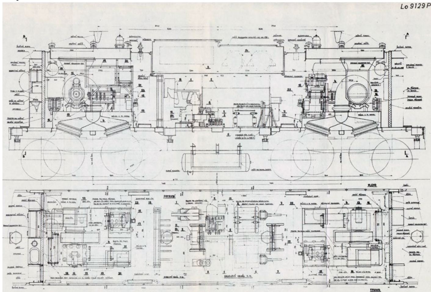
▲ Bokorys a půdorys znázorňující rozmístění výzbroje ve strojovně lokomotivy.
