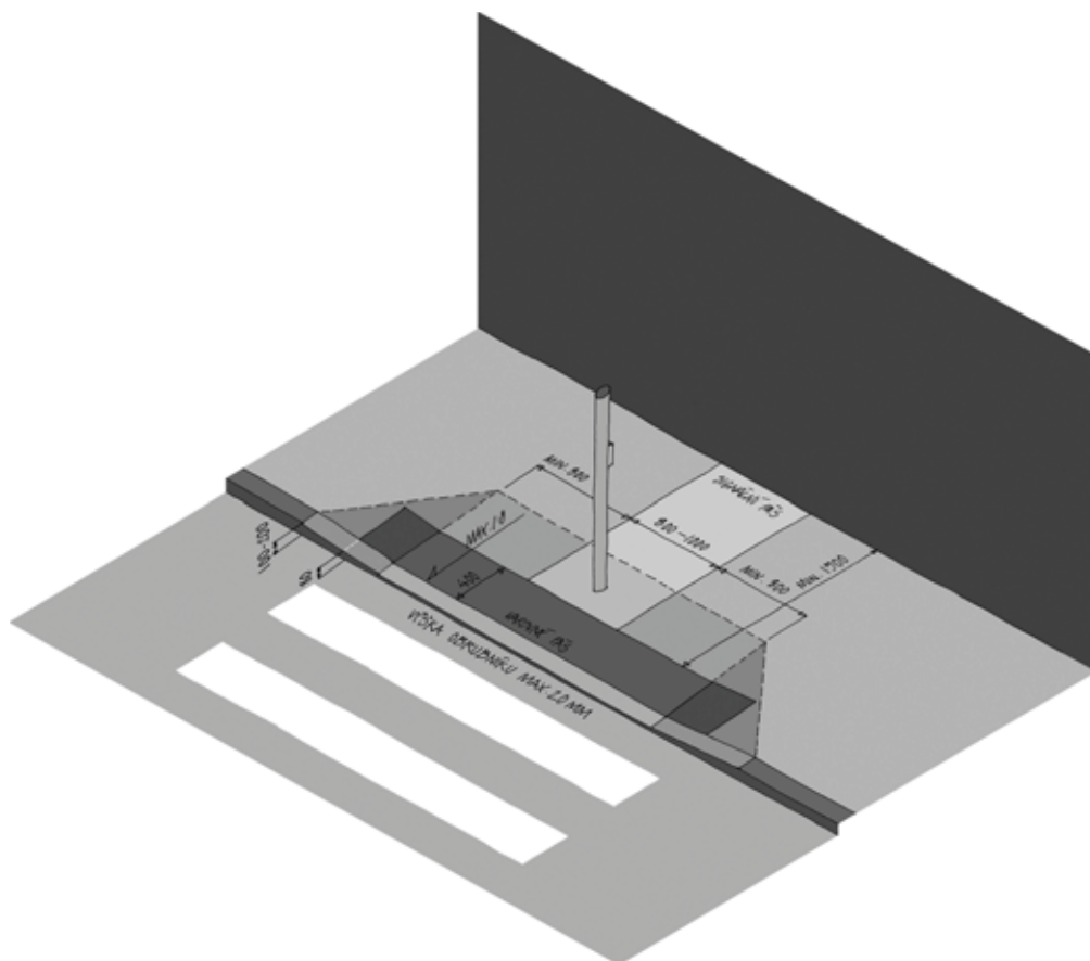
Obr. 2.1 Přejezd pro chodce – detail
