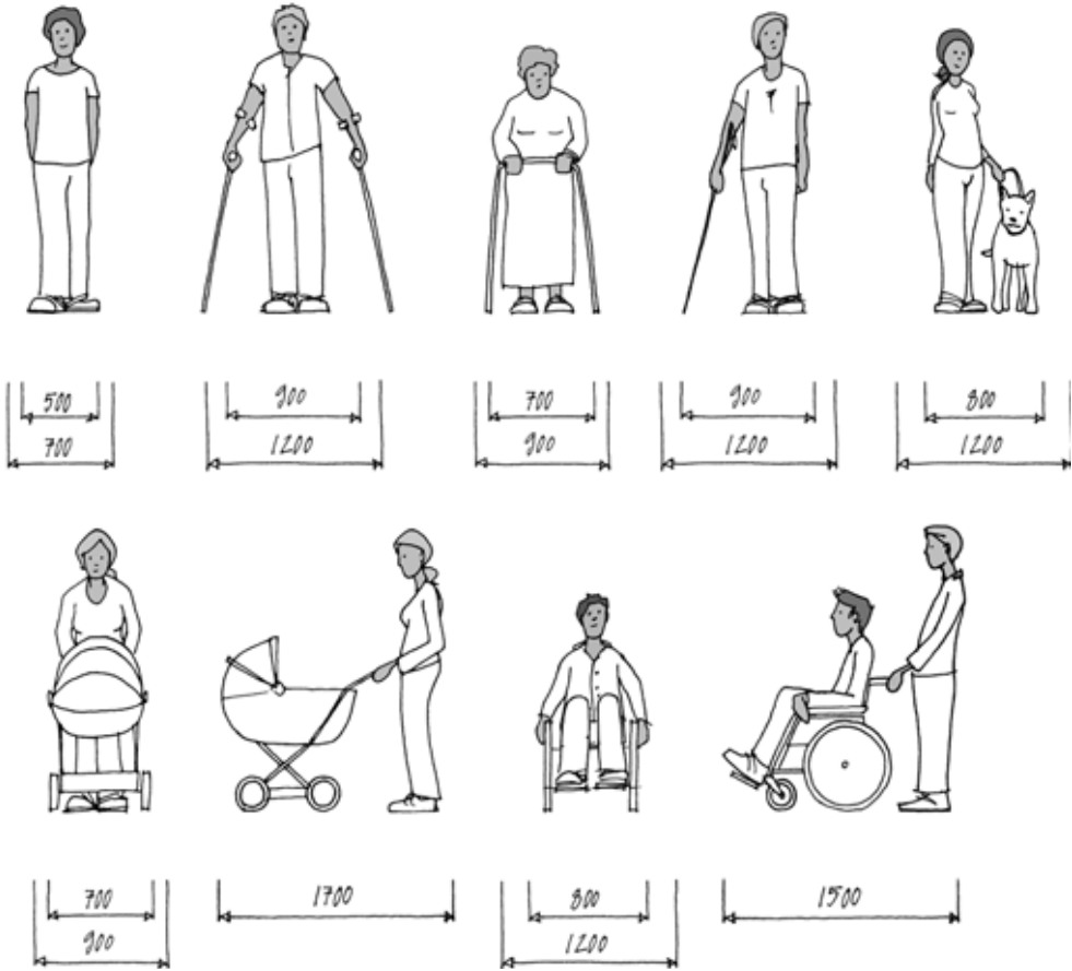
Obr. 1.3 Prostorové požadavky – osoba bez opory, osoba o berlič, osoba s chodítkem, nevidomý, nevidomý se psem, osoba s kočárkem, vozičkář, vozičkář s asistencí
